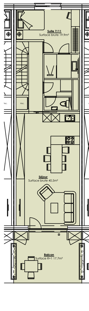
Maison 7 Surface brute R+1 77.5m 2
