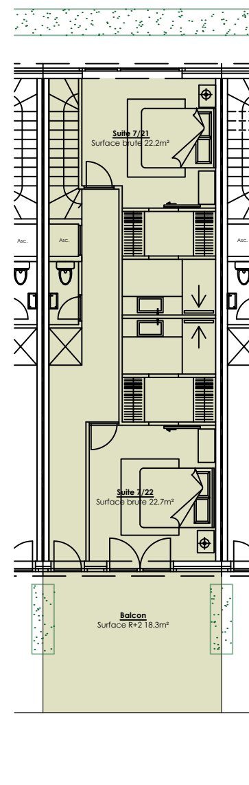
Maison 7 Surface brute R+2 66.5m 2
