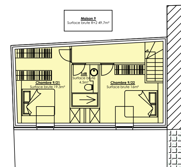
Plan R+2
